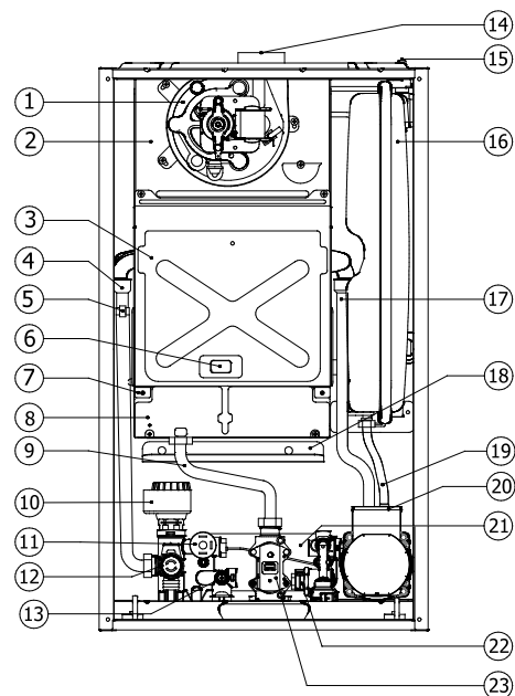
Рисунок 25. Компоненты котла
