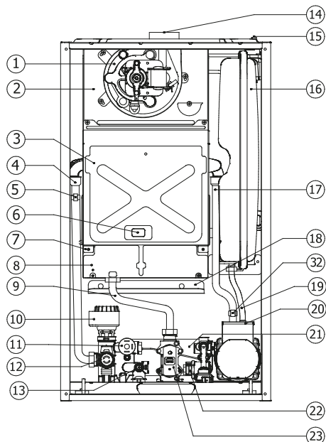
Рисунок 38 Компоненты котла
