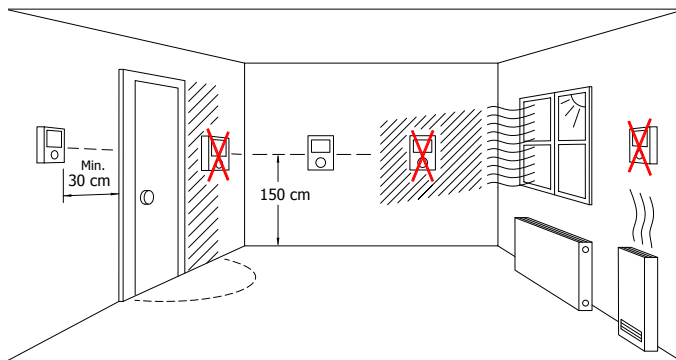
Рисунок 45 Положение термостата
