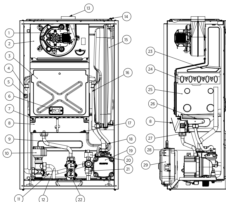
Рисунок 25. Компоненты котла
