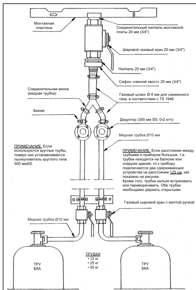
Рисунок 9 Подключение газовой трубы котла, если длина шланга более 125 см
