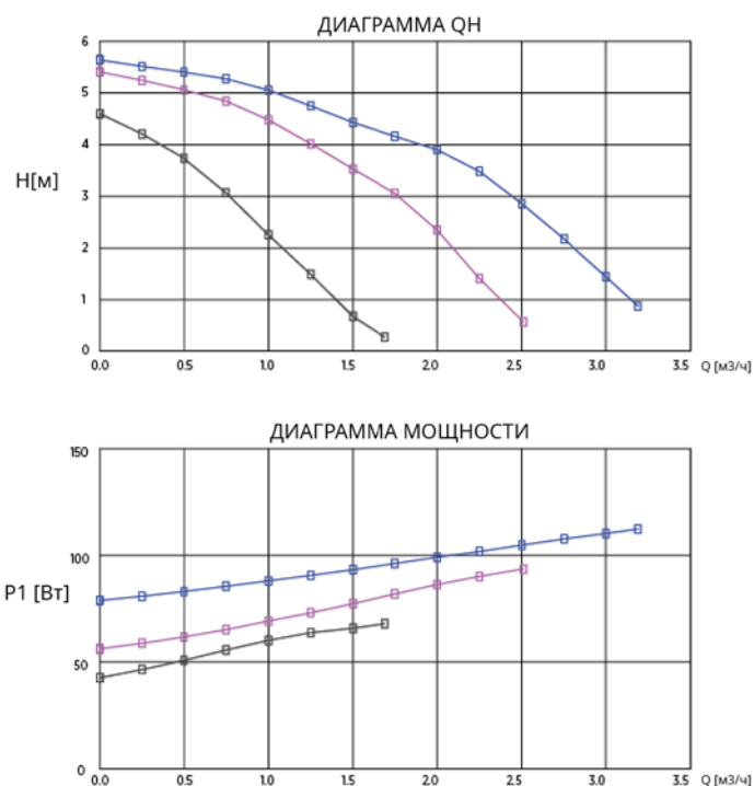
Рисунок 27 График расхода / давления насоса
