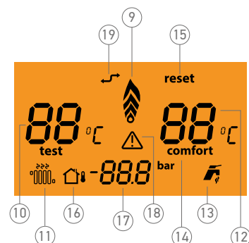
Рисунок 42 Экран автоматической панели управления Lawa Plus
