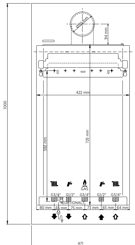
Рисунок 1 Монтажный шаблон
