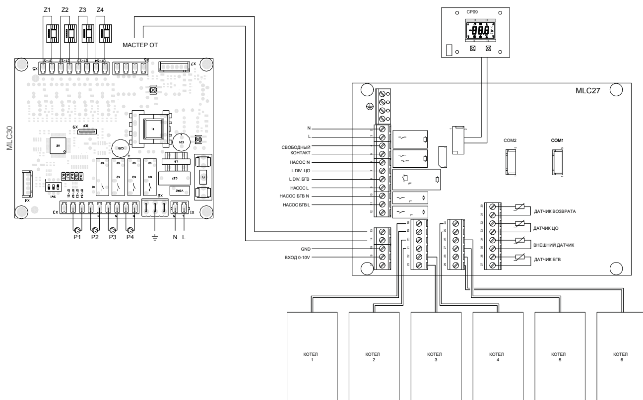
Рисунок 36 Схема электрических соединений MLC 27 и MLC30 для Lawa System / Lawa Plus System / Lawa Pro System с каскадной системой и 4 зонами высокой температуры (радиаторы)
