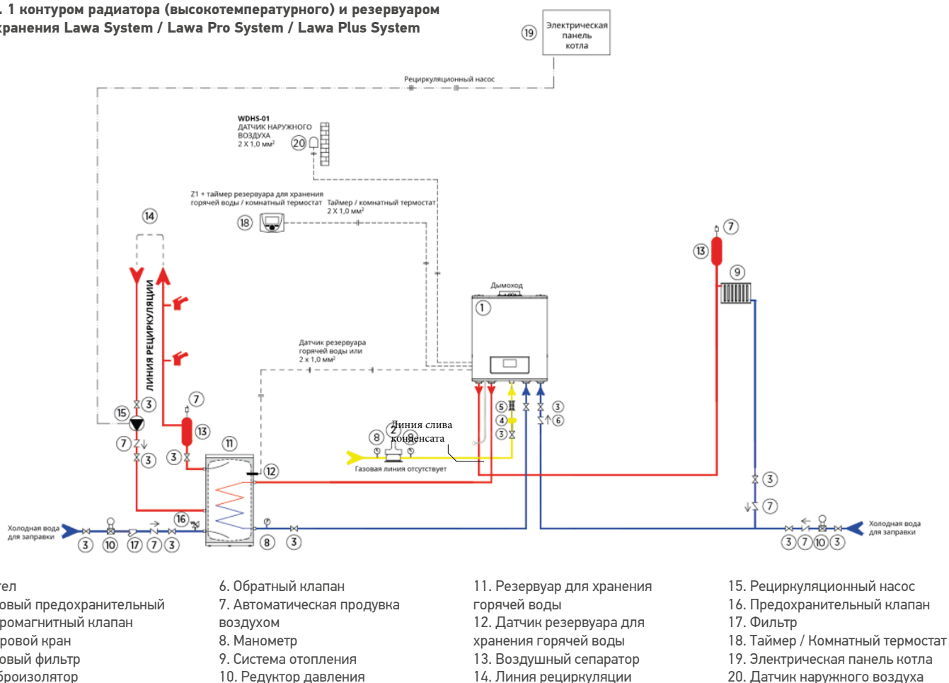
Рисунок 34 Схема системы с одним котлом Lawa System / Lawa System / Lawa Pro System (1 HT + бак для хранения горячей воды)
