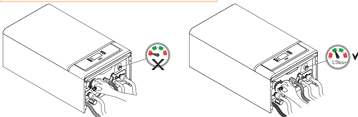
Рисунок 24 Подача водопроводной воды отопителя через заправочный клапан котла и контроль давления.
