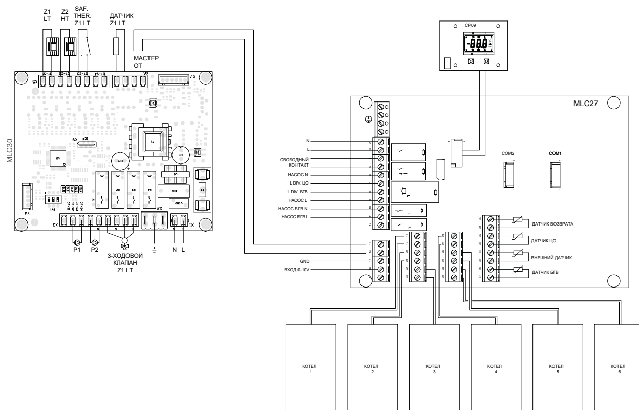
Рисунок 37 Схема электрических соединений MLC 27 и MLC30 для котлов Lawa Plus System / Lawa Pro System с каскадной системой и 1 зоной низкой температуры (теплый пол)
